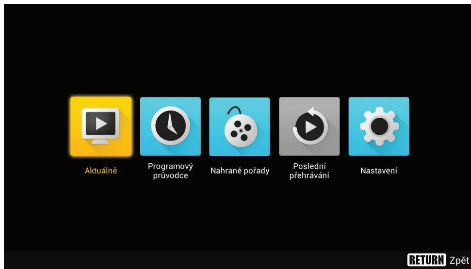
Obrázek 4: Hlavní menu
